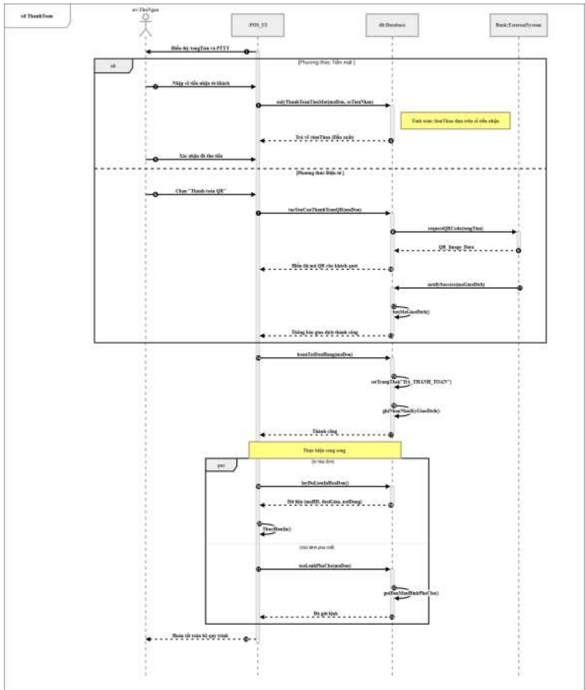
Hình 2.7 Sơ đồ Sequence Thanh toán
