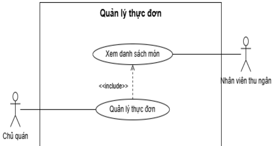
Hình 2.4 Sơ đồ UseCase Quản lý thực đơn
