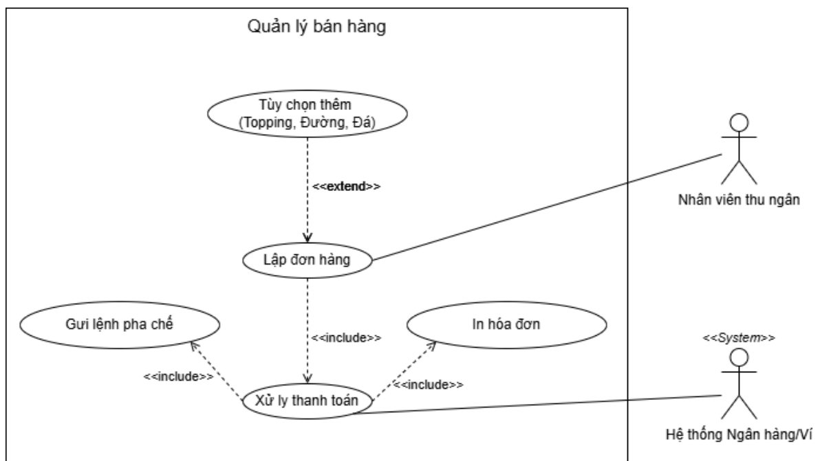
Hình 2.2 Sơ đồ UseCase Quản lý bán hàng
