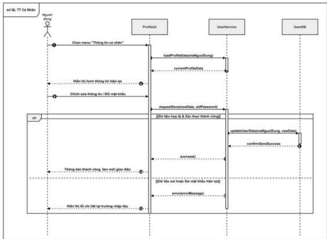
Hình 2.11 Sơ đồ Sequence Quản lý thông tin cá nhân
