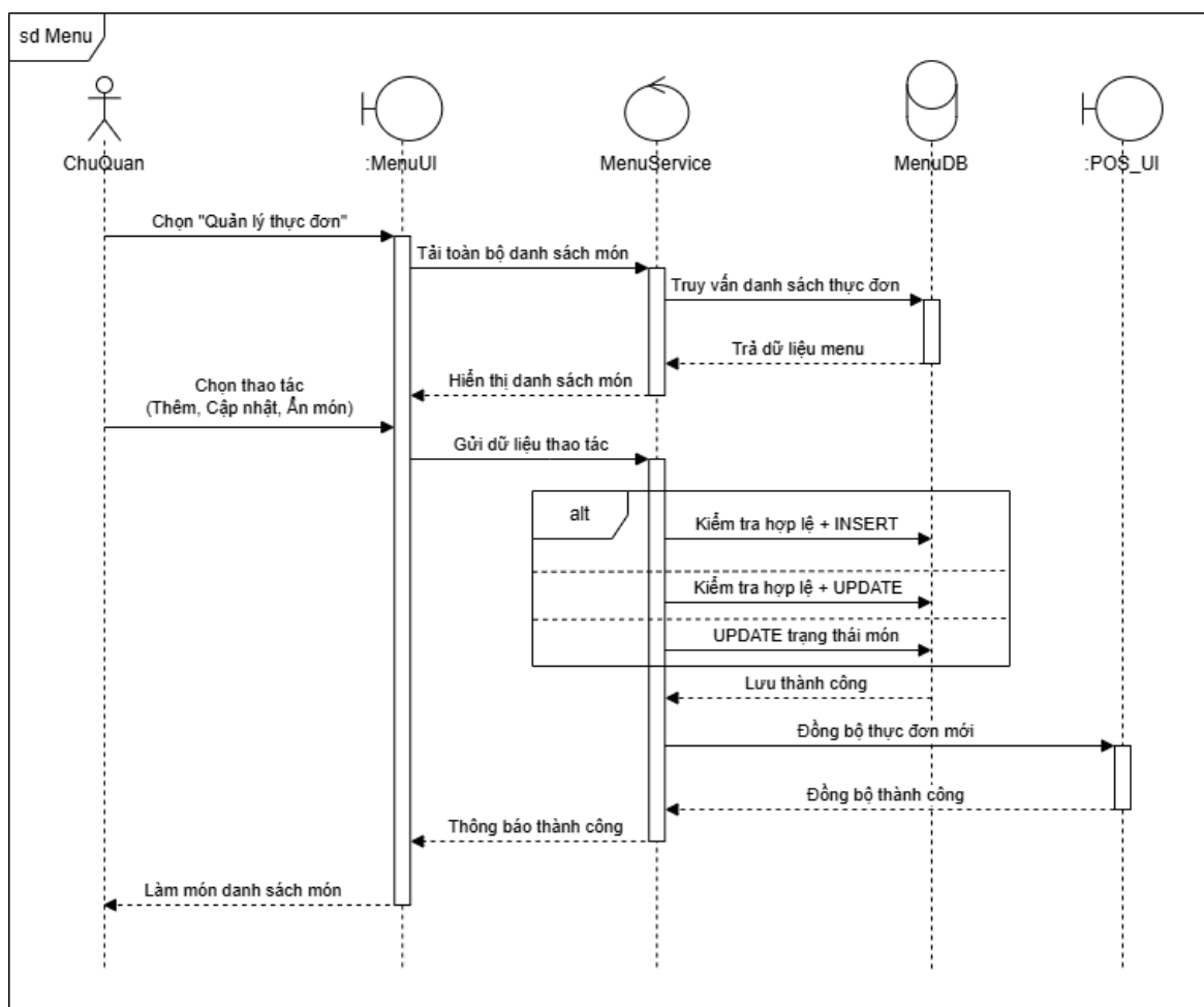
Hình 2.10 Sơ đồ Sequence Quản lý thực đơn
